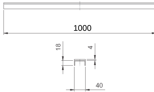
Abdeckung Design (4 mm Edelstahl)
